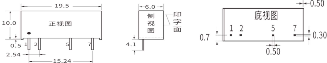
2)引脚定义
